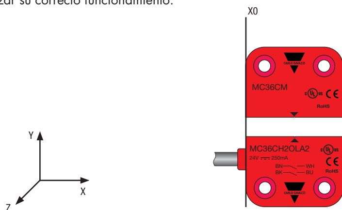
Fig. 2 - Sentido de alineación y funcionamiento de los sensores
