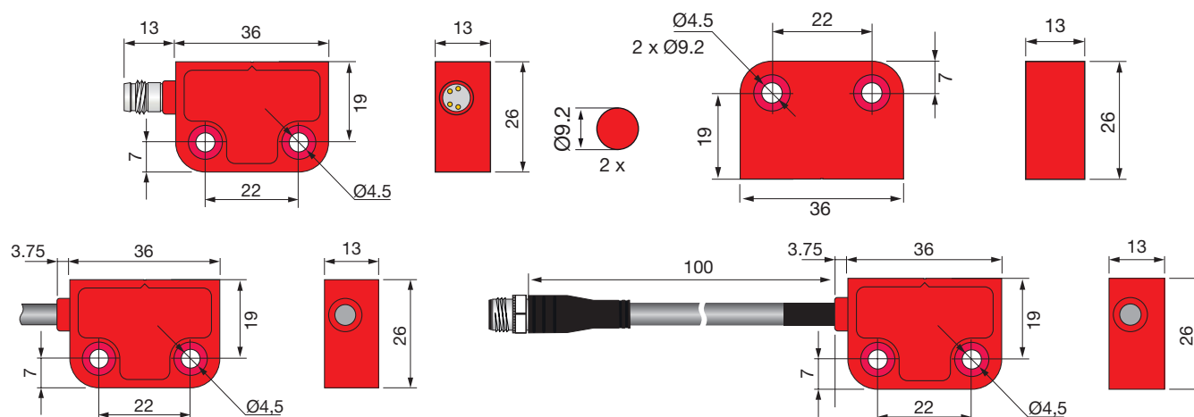
Fig. 1 - Dimensiones
