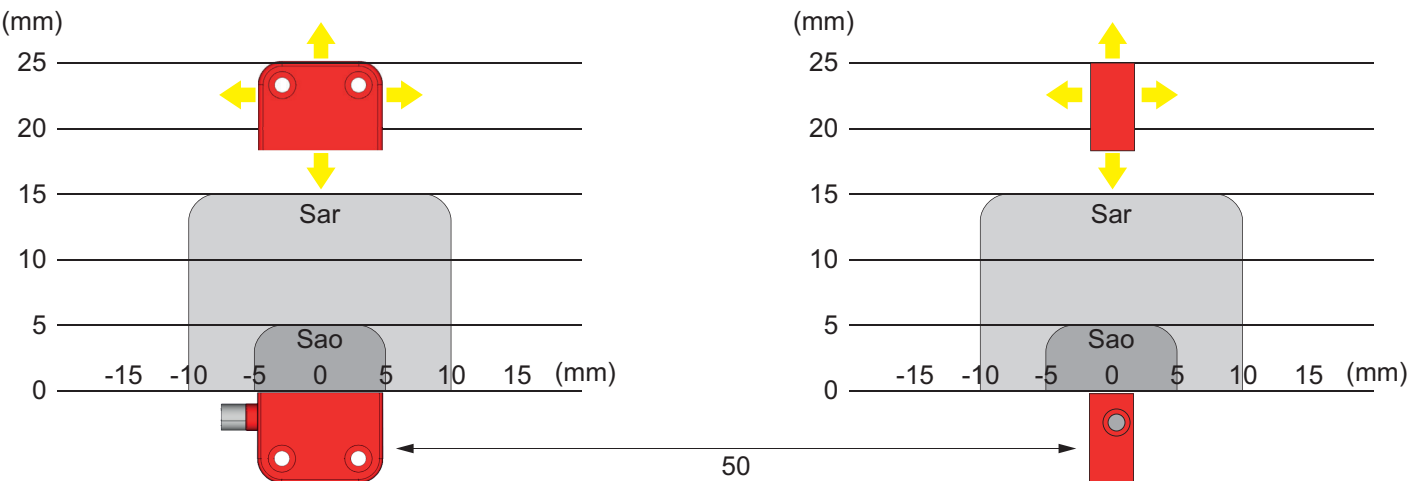
Fig. 3 - Distancia
