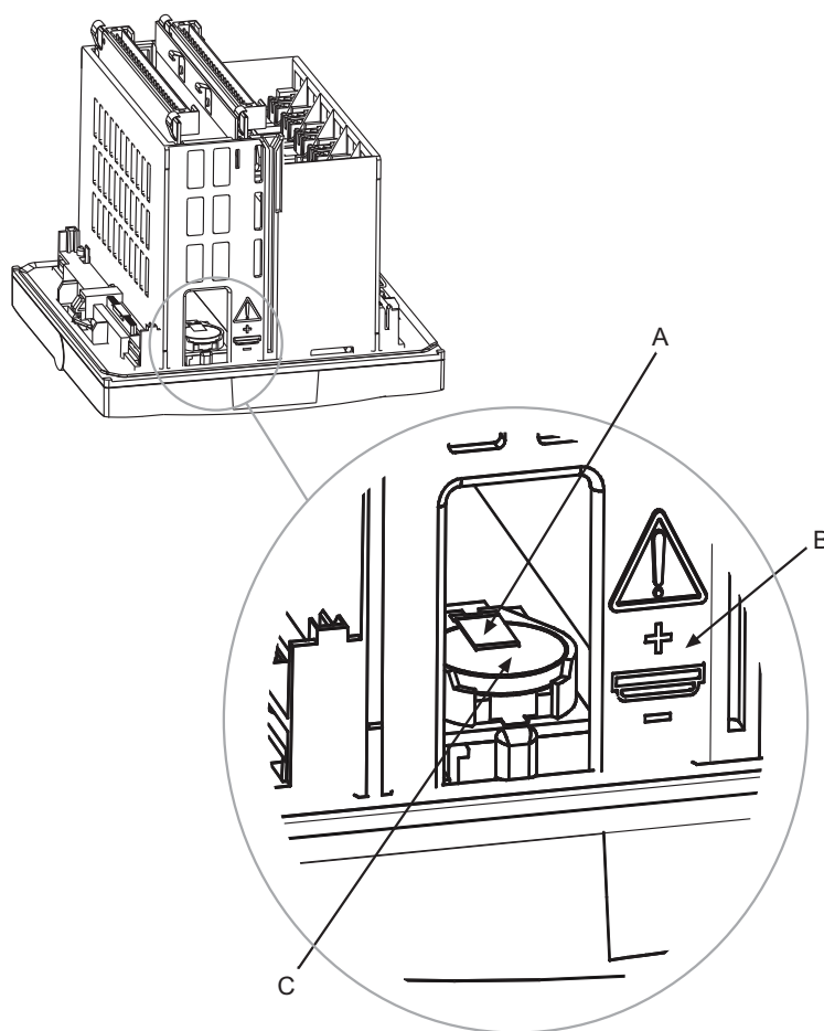
Fig. 4.4.3.-1 Insertar y cambiar la batería
