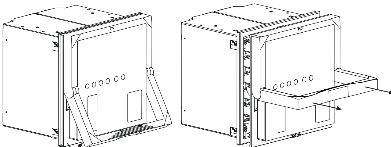
Fig. 4.4.2.-1 Desconexión de una unidad central de la caja
