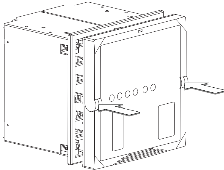
Fig. 4.4.2.-2 Instalación de una unidad central en la caja
