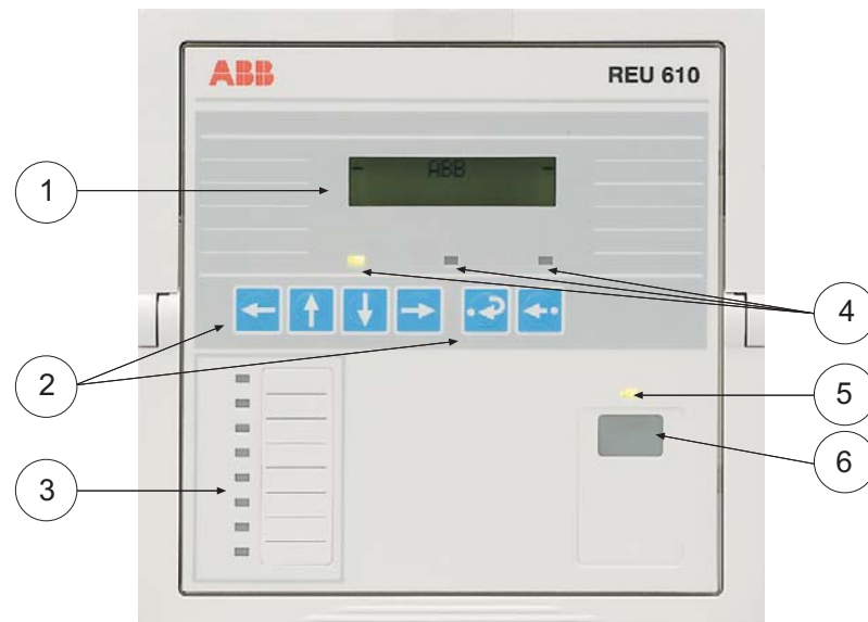
Fig. 4.1.1.-1 Vista frontal del relé
