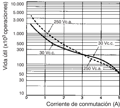
MY4 (Cargas resistivas)
