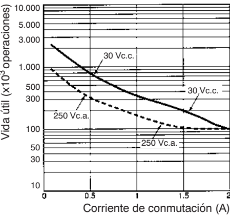
MY4 (Cargas inductivas)
