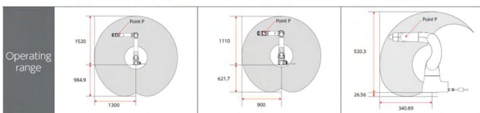
COBOTTA PRO 1300
