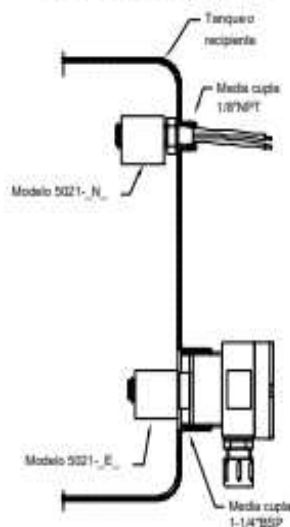
MONTAJE TÍPICO PARA LLENADO O VACIADO.
