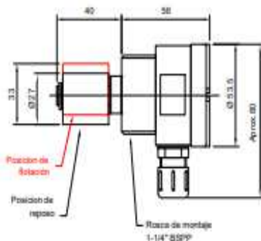
Modelo 5021- _E_ (montaje exterior)
