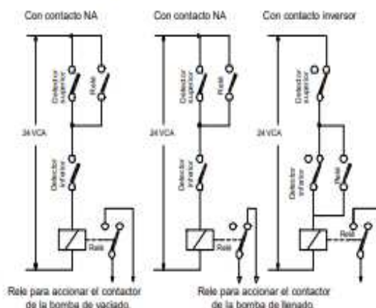
MONTAJE TÍPICO PARA LLENADO O VACIADO.
