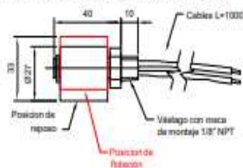
Modelo 5021- _N_ (montaje interior)
