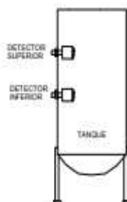
MONTAJE TÍPICO PARA LLENADO O VACIADO.
